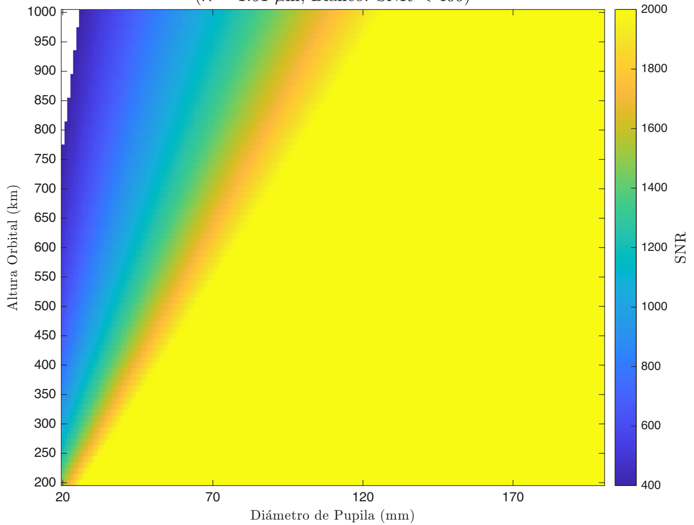
SNR - TMA - Detector 3 ( \lambda = 1.61 \mu\text{m} , Blanco: SNR < 400)
